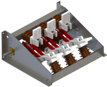
MI-COMP-CI 3,6-5kV 2000A Manual
