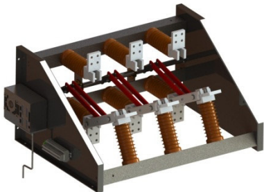
MI-COMP-CI 24kV 2600A + Motor M
