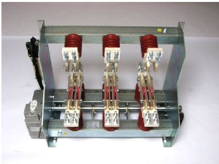
MI-COMP-CI 12kV 2500A + Motor M
