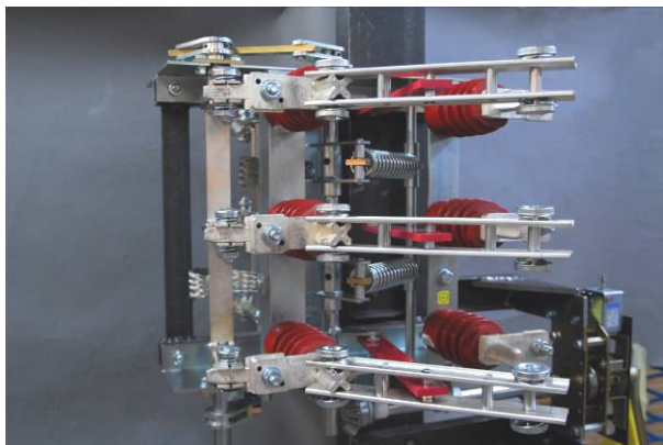
MIT 12kV 400A 3p + CDZ1
